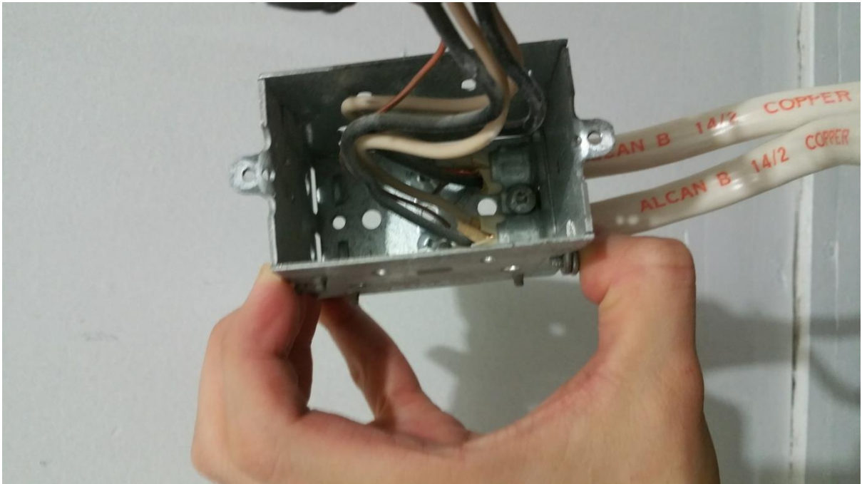
제거한 콘센트 2
